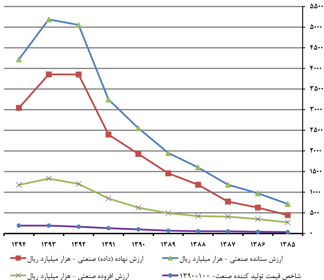
نمودار ۷- روند ارزش نهاده (داده)، ستانده و افزوده‌ی صنعتی کارگاه‌های صنعتی ۱۰ نفر کارکن و بیش‌تر و شاخص قیمت تولید کننده صنعت در سال‌های ۱۳۸۵-۱۳۹۴
